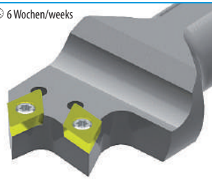
Beispiel: ISO Platten auf Sonderbohrstangen Example: ISO inserts on special boring bars
