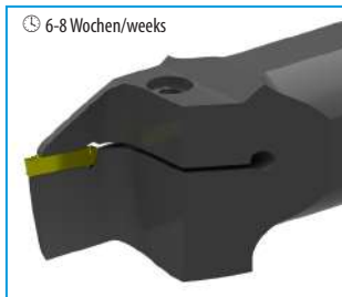
Beispiel: Innenaxialbohrstange Example: internal face-grooving boring bar
