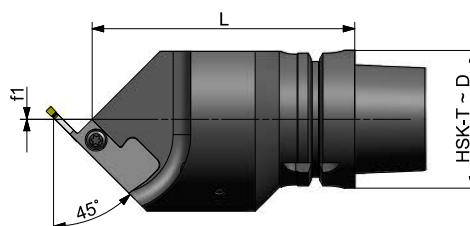
GLM HSKT 45 R
