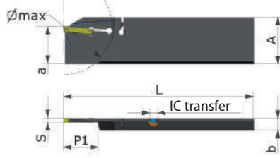
P92 CXCB R 3208X... R/L65HP
