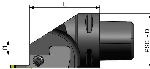
GLM PSC 0 L
