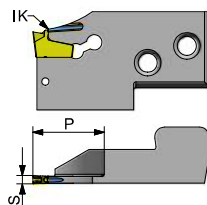
GLM CL F16...HP
