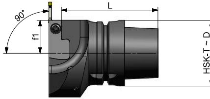
GLM HSKT 90 R
